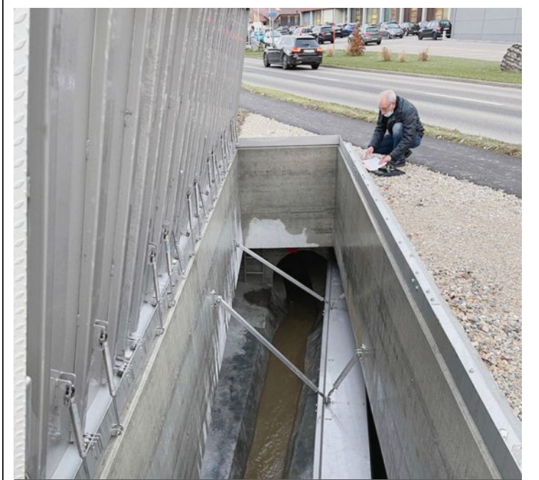
Le nouveau dégrilleur à l'entrée est du village.
